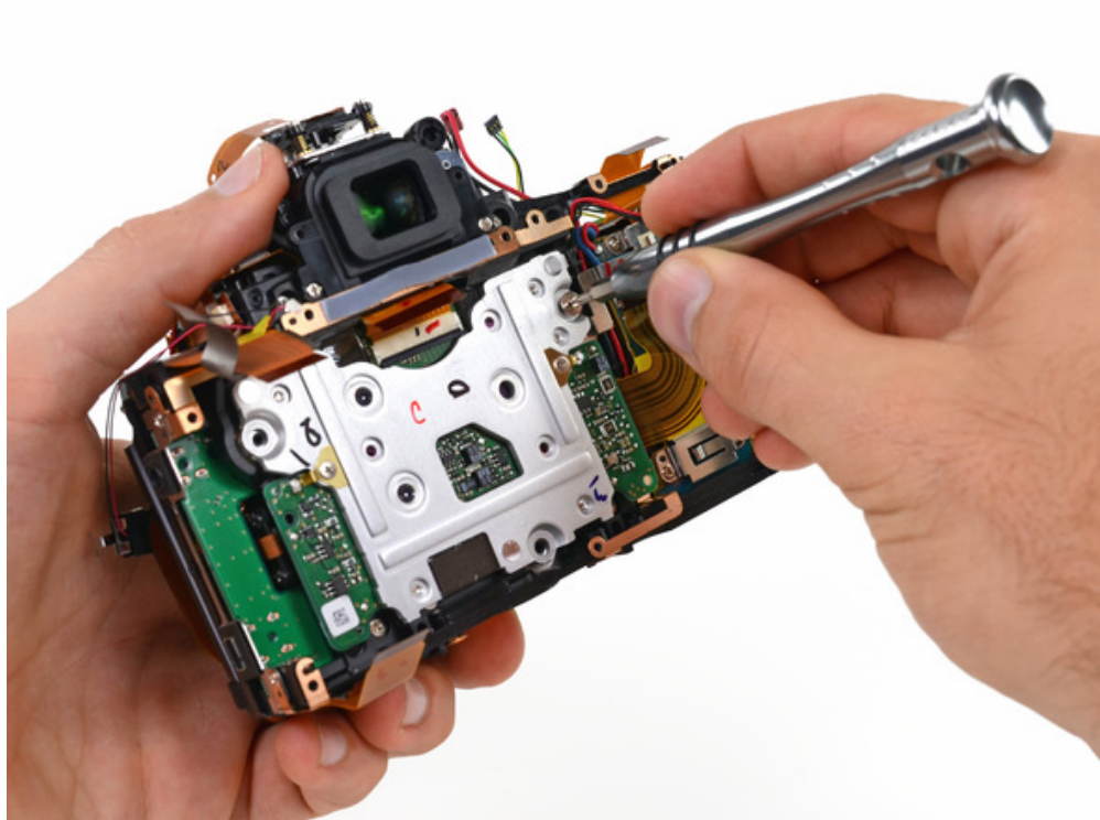
Démontage de la face arrière du Nikon D600 après retrait de l'écran LCD
