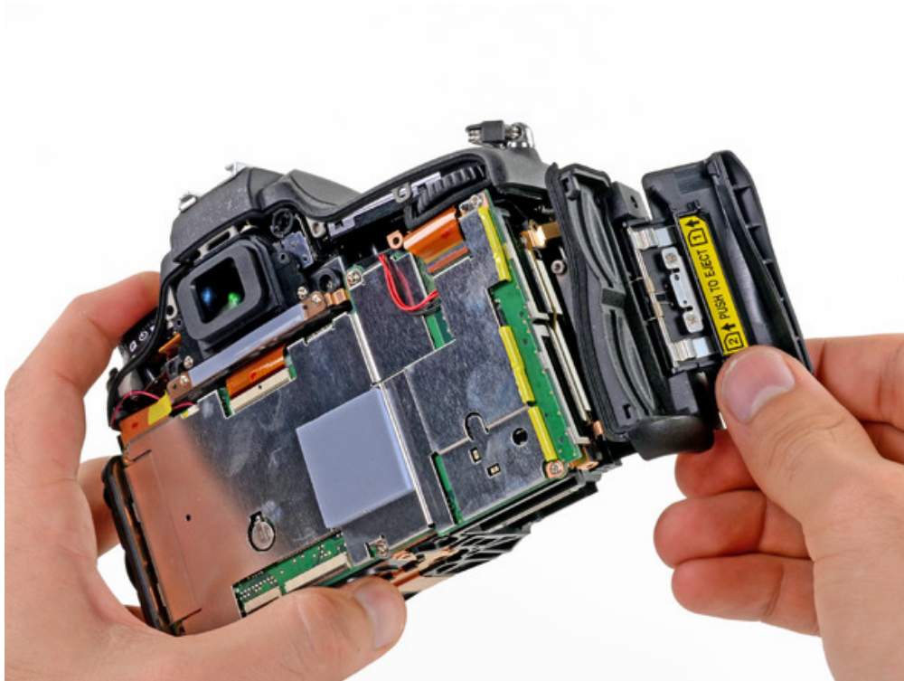
Démontage des éléments latéraux et du boîtier du Nikon D600
