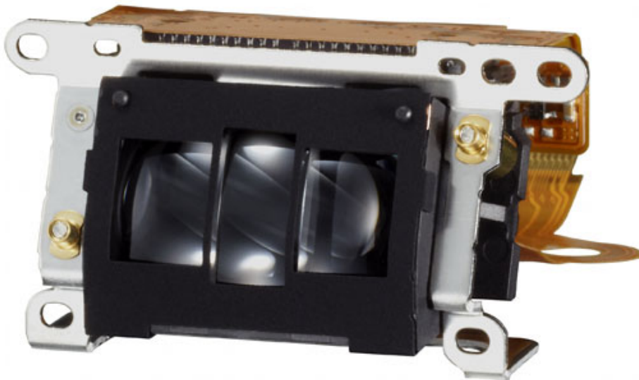
Le module autofocus du Canon 5D Mark III
