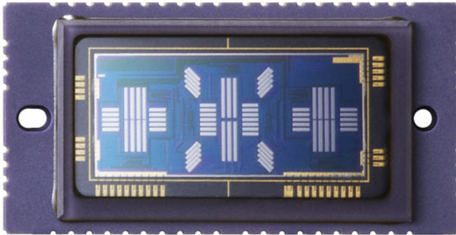
Le capteur autofocus du Canon 5D Mark III
