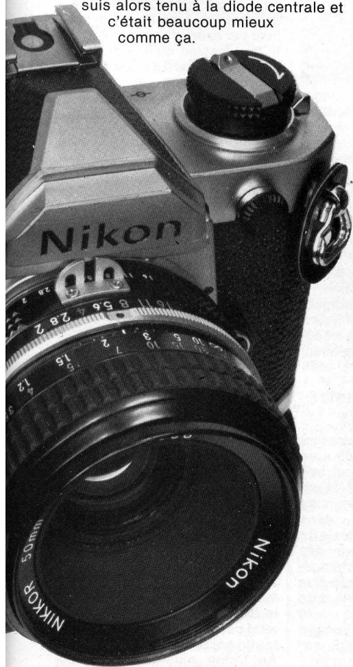
La conception traditionnelle de Nikon FM se retrouve dans la disposition de ses organes extérieurs. A remarquer cependant le sélecteur « déclenchement moteur-déclenchement normal » autour du déclencheur, la petite plaque de cuir qui protège l'appareil des cavaliers et, caché derrière le sélecteur de vitesses, le bouton de surimpression.
